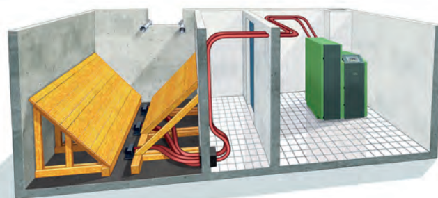
Trois à huit sondes permettent d'exploiter chaque silo de stockage de manière optimale.
